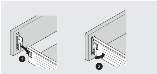
Reelingin asennus
