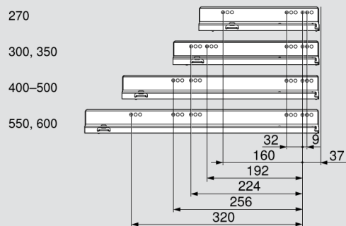
Runkokiskojen mitoitus
