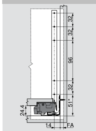
Etulevynmitoitus ruuvi
