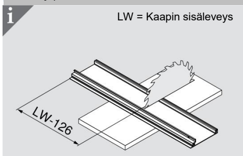
Etusarjaprofiili
