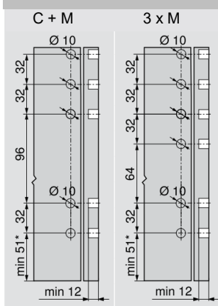
Etulevynmitoitus EXPANDO
