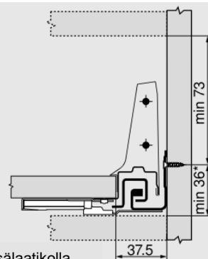
Tilantarve M -sisälaatikolla
