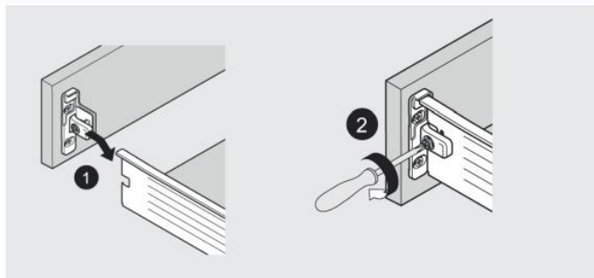
Sisälaatikko 320M/H
