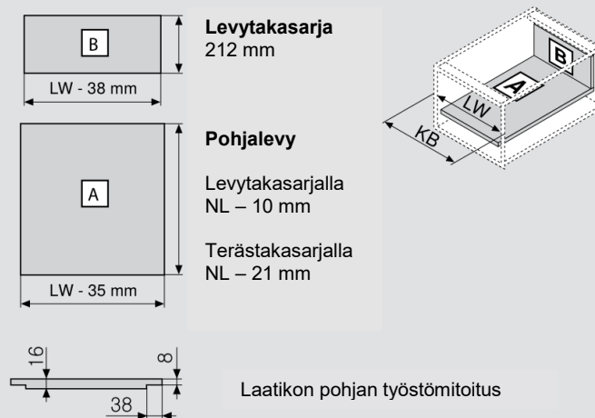
Laatikon pohjan ja levytakasarian mitoitus 16 mm melamiinilevyllä
