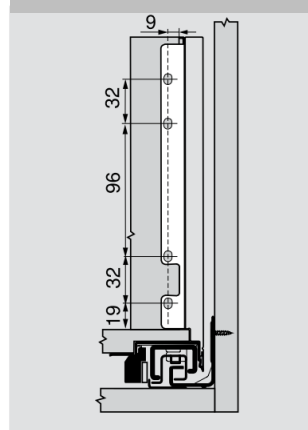
Levytakasarin mitoitus
