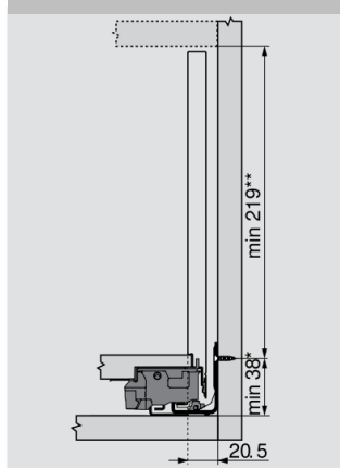
Tilantarve kaapissa
