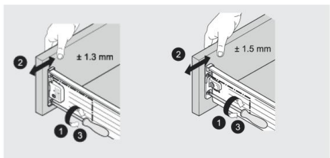
Sivusäätö M/H
